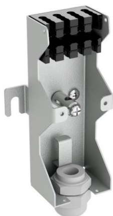
Widok wnętrza rozdzielacza tub
