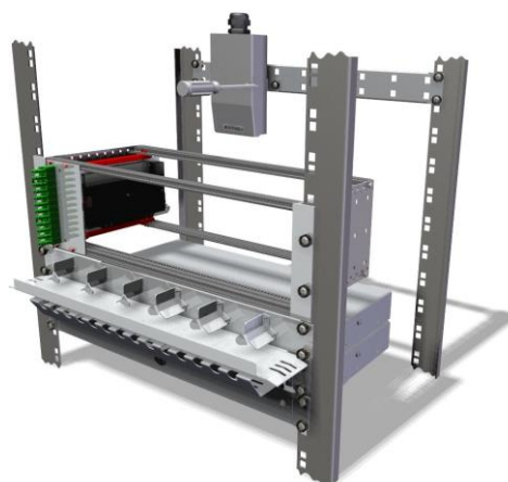
Widok zamontowanego rozdzielacza tub na listwie rozdzielaczy
