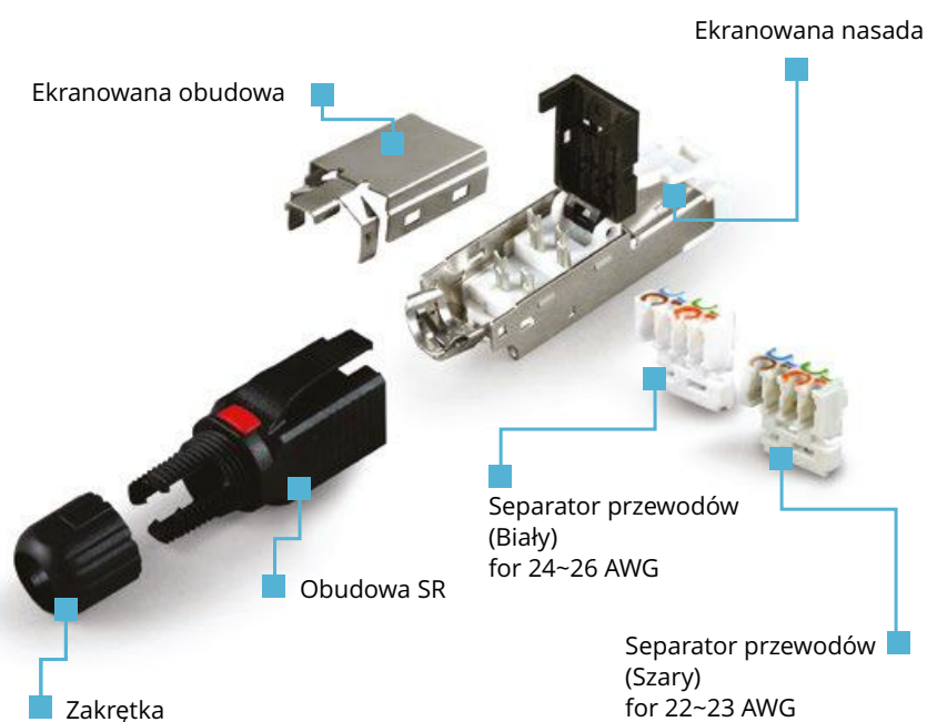
Rysunek 1. Schemat budowy beznarzędziowych RJ45
