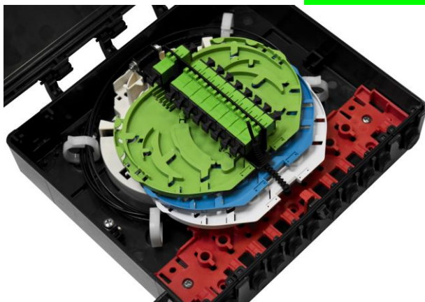
Widok wnętrza mufoprzełącznicy w wersji OBP-S8.
