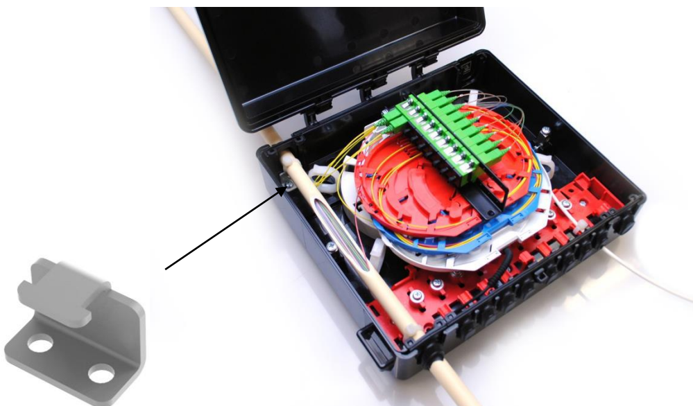
Widok przykładowo wyposażonej mufoprzełącznicy w wersji OBP-S8 z zamocowanym uchwytem kabla wewnątrzbudynkowego.
